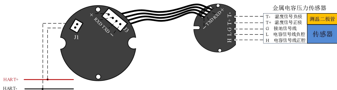
图 2.3 HART 电容压力套卡接线示意图
