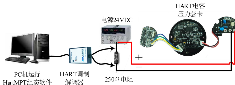
图 2.4 系统连接示意图
