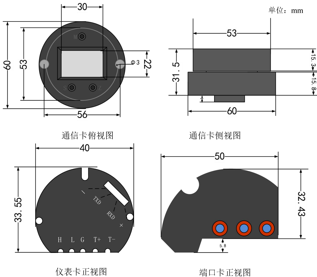
图 2.1 MS0010 HART 电容压力套卡尺寸
