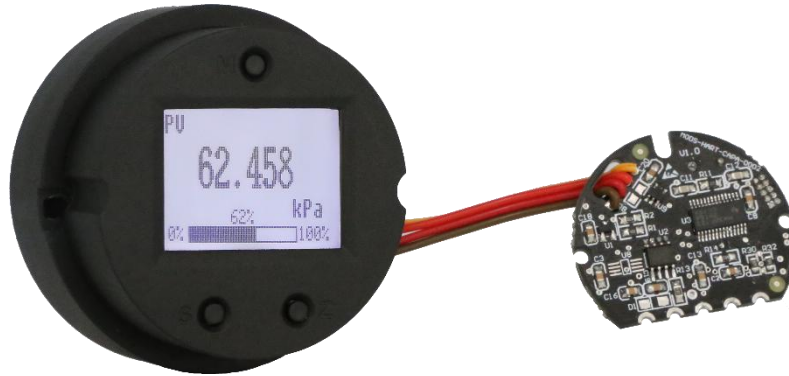
图 1.1 MS0010 HART 电容压力套卡
