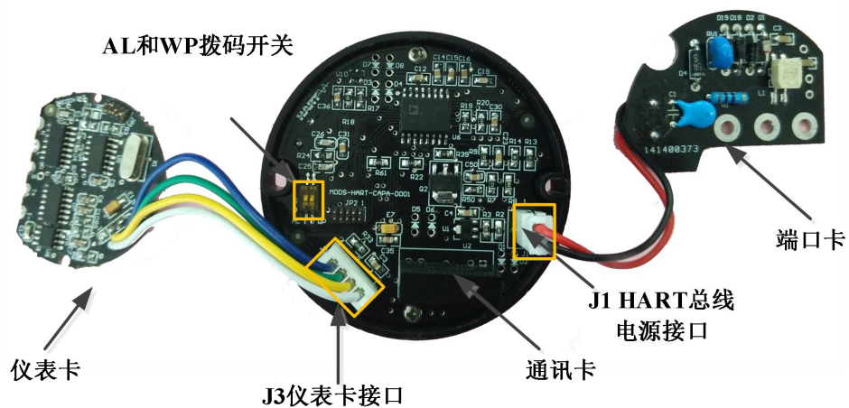
图 2.2 硬件接口说明
