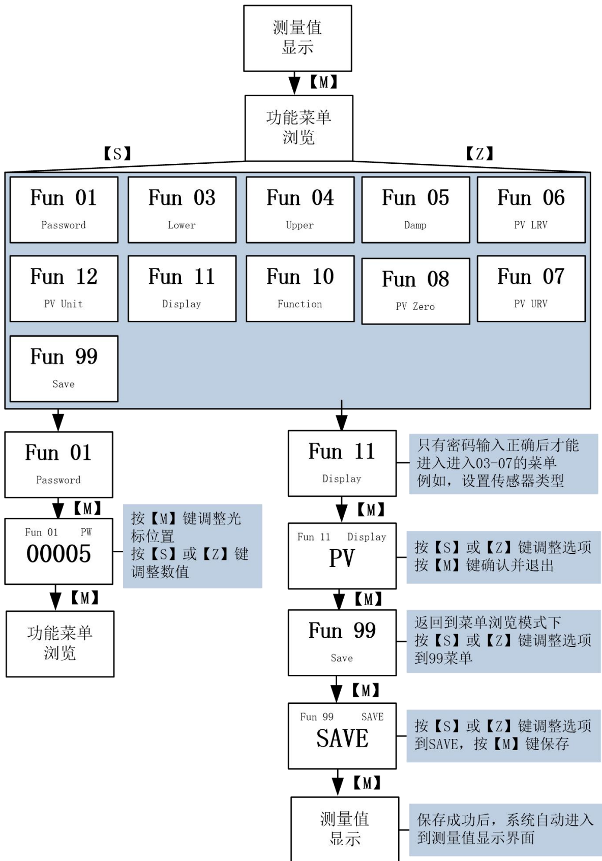
图 15 功能切换图
