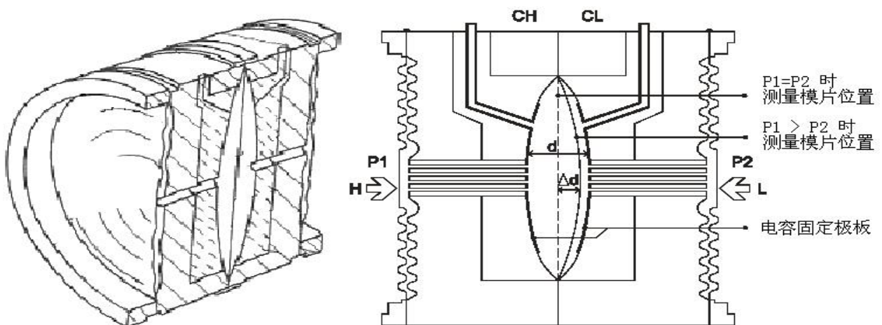
图 3.2 传感器电容膜盒
